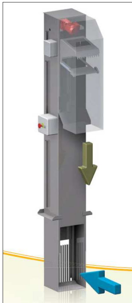
Dégrilleur vertical de Petite-Chapelle (SG 400 – FBPROCEDES)
